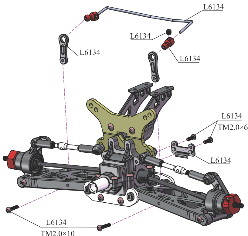
L6134 TM2.0×10mm
