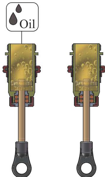
L6115/L6121 SØ 5.8
