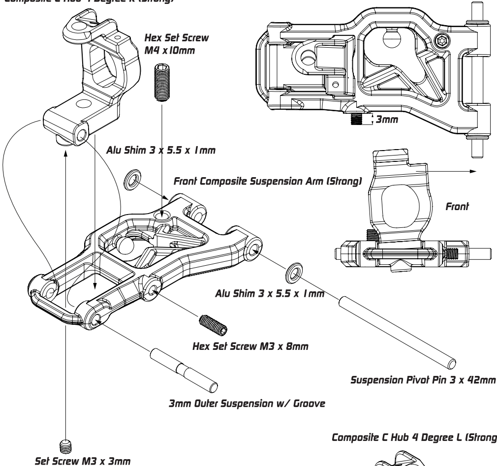
Strong Front Composite Suspension Arms V2 XP-10923
