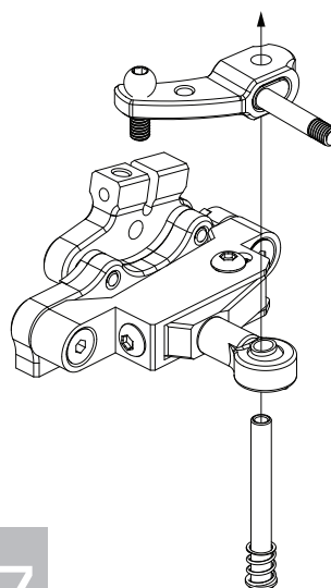
Front Spring (Medium/Gold) C-02-VBC-5042 x 2
