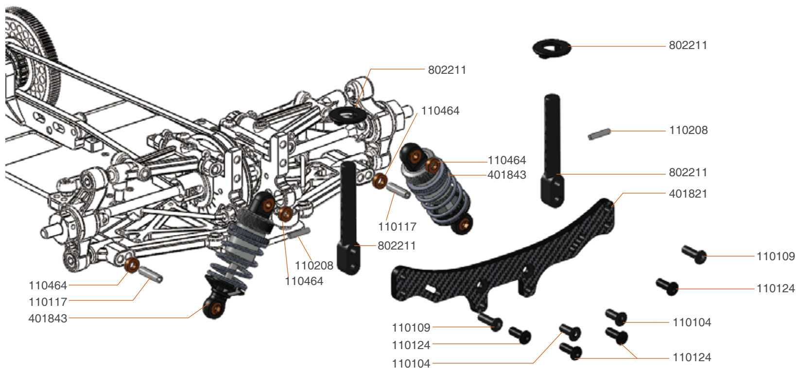
401843 Shockset (2) X20
