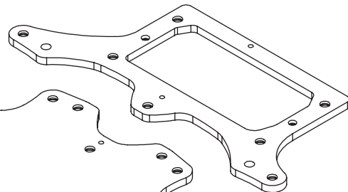
220164 2.5mm Graphite Lower Pod グラファイトロアブレース
