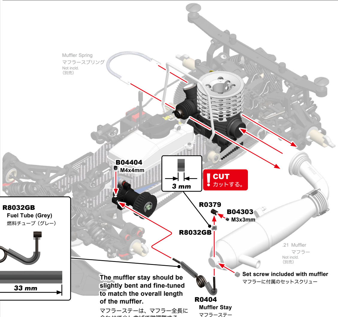
SMJ1374 SMJ Kabuto Tuned Silencer Set Spec 3 (for 1/8 Racing) SMJ Kabuto チューンドサイレンサーセット スペック 3 (1/8 レーシング)
