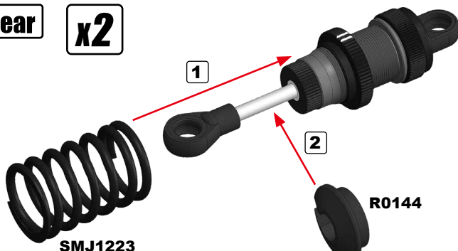
Stealth Line Spring RL5.0 (Long 27mm) ステルスラインスプリング (ロング)
