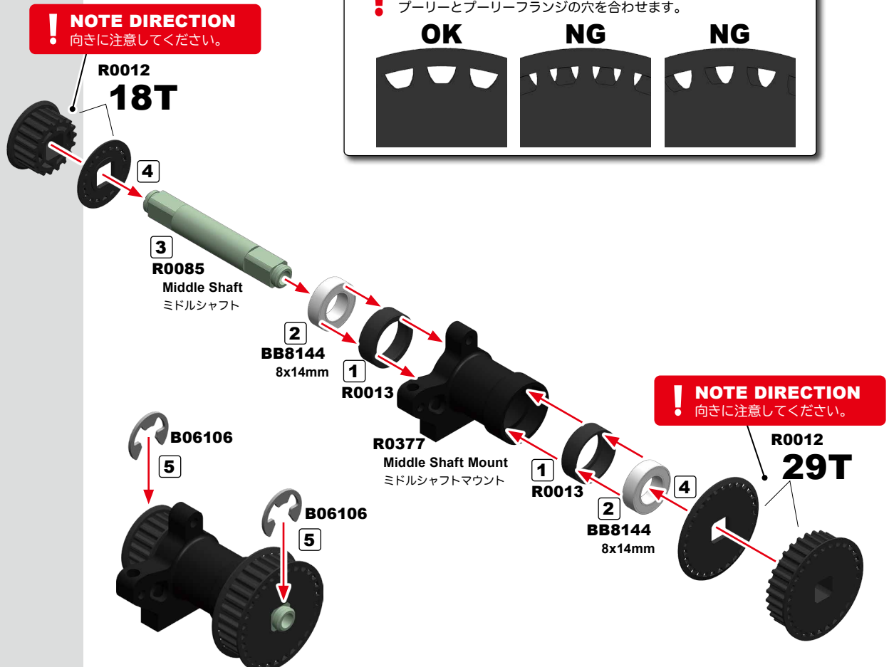
BB8144 Ball Bearing 8x14mm ボールベアリング
