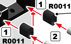
R0230-IN Rear Lower Sus Holder 7075 IN リア ロアサスホルダー 7075 (IF18) イン
