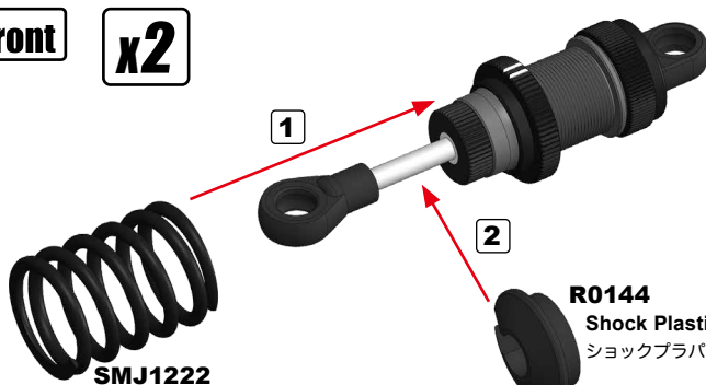
Stealth Line Spring RS8.6 (Short 24mm) ステルスラインスプリング (ショート)
