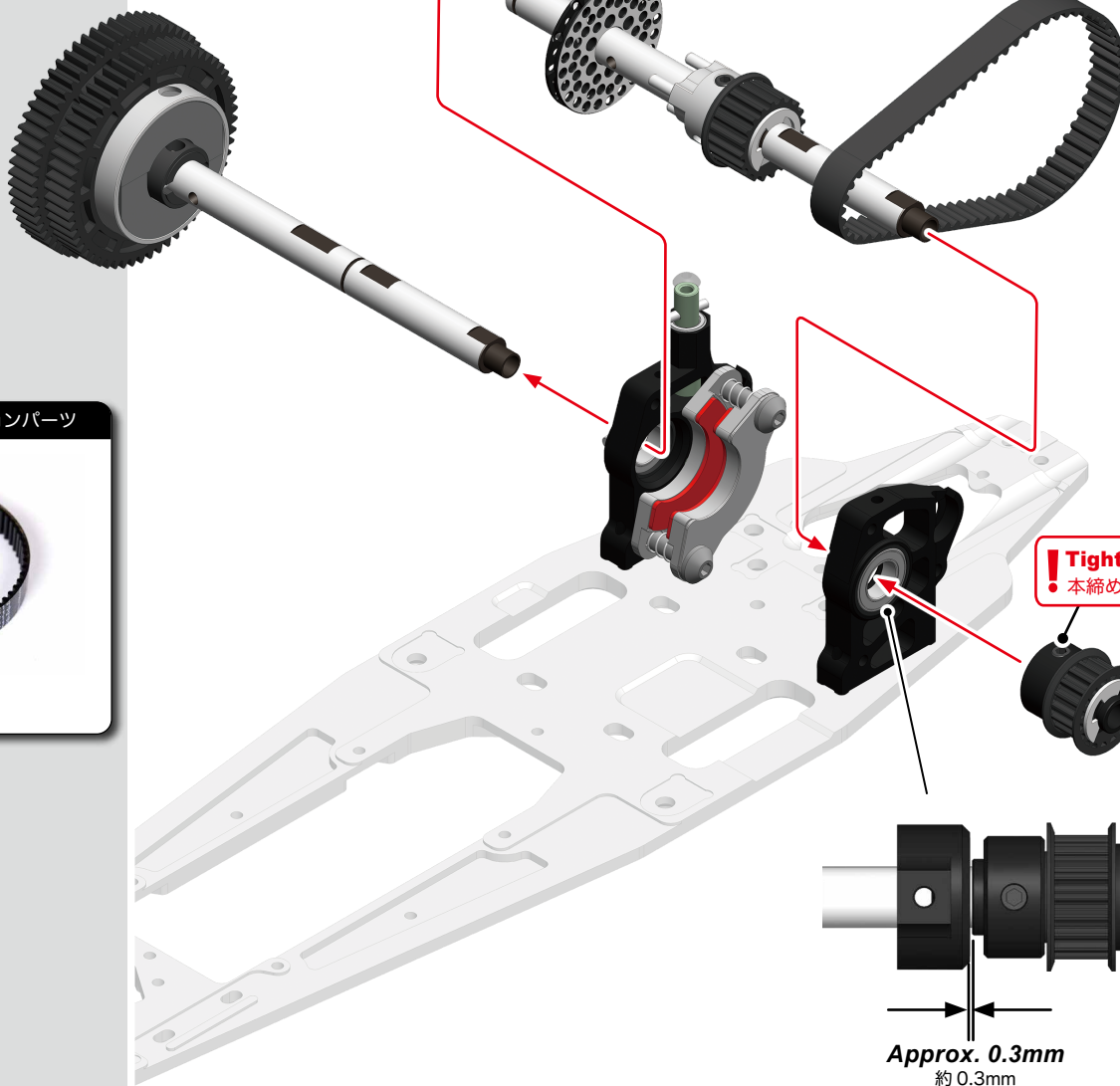
R8009B Rear Belt (Urethane) 201 リアベルト (ウレタン) 201
