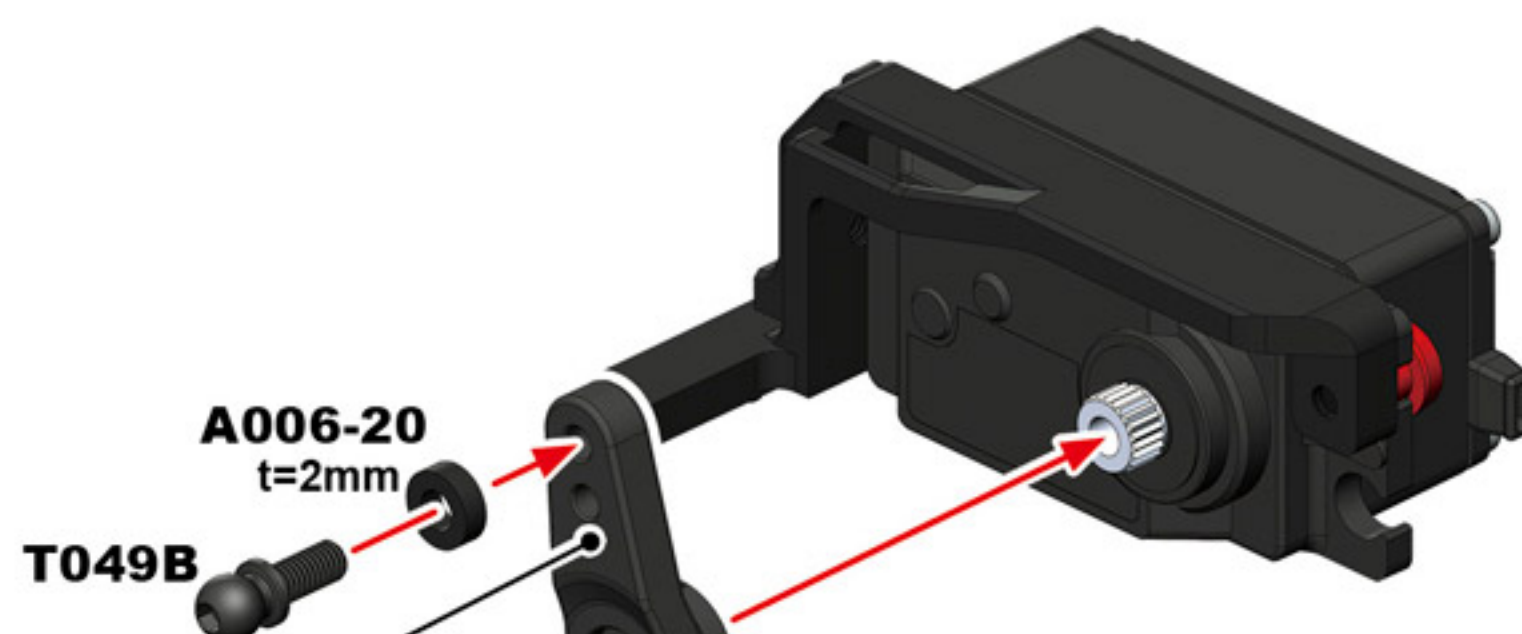
T007 Servo Horn, Steering Arm Set サーボホーン, ステアリングアームセット
