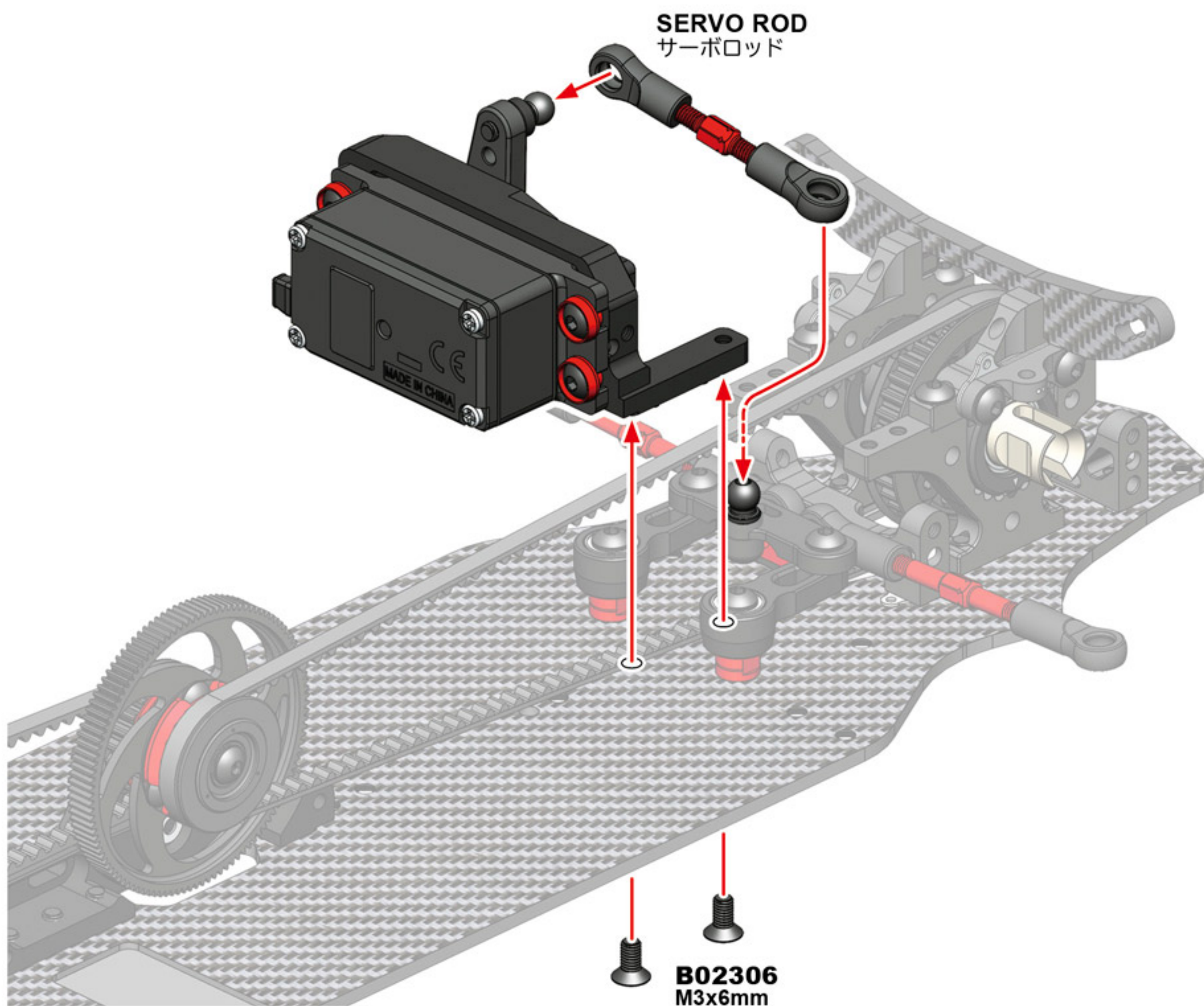
T091 Alu Adjustable Servo Horn (for Sanwa) アルミアジャスタブルサーボホーン (サンワ用)
