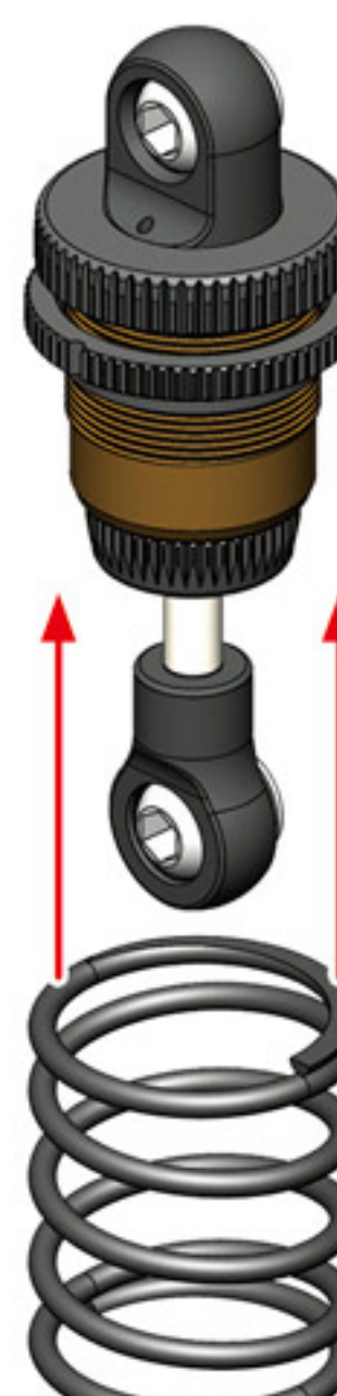
SMJ1242 Stealth Line Lefty Spring TS2.7 ステルスラインレフティスプリング
