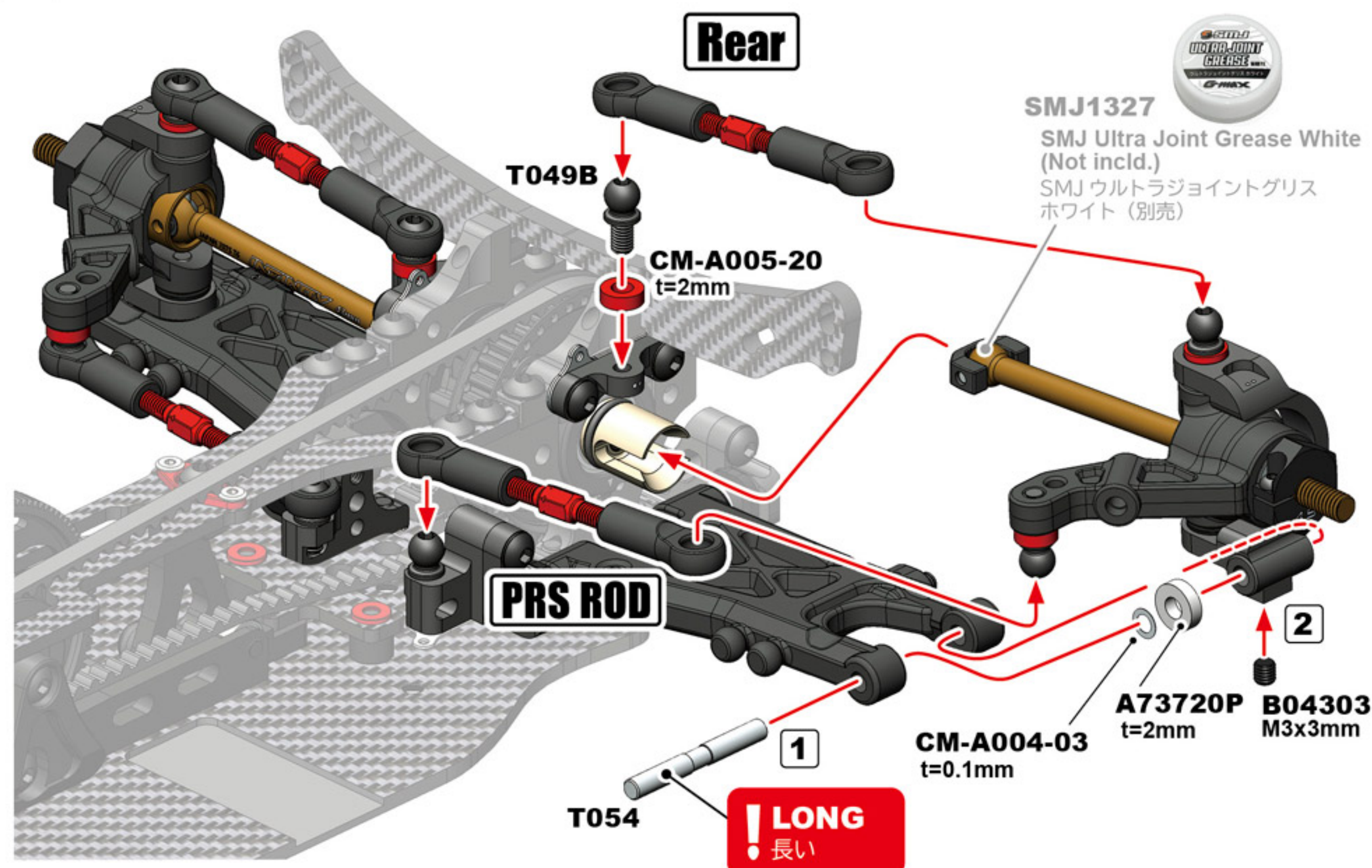
B04303 M3x3mm Set Screw (Cup Point) セットスクリュー (くぼみ先)
