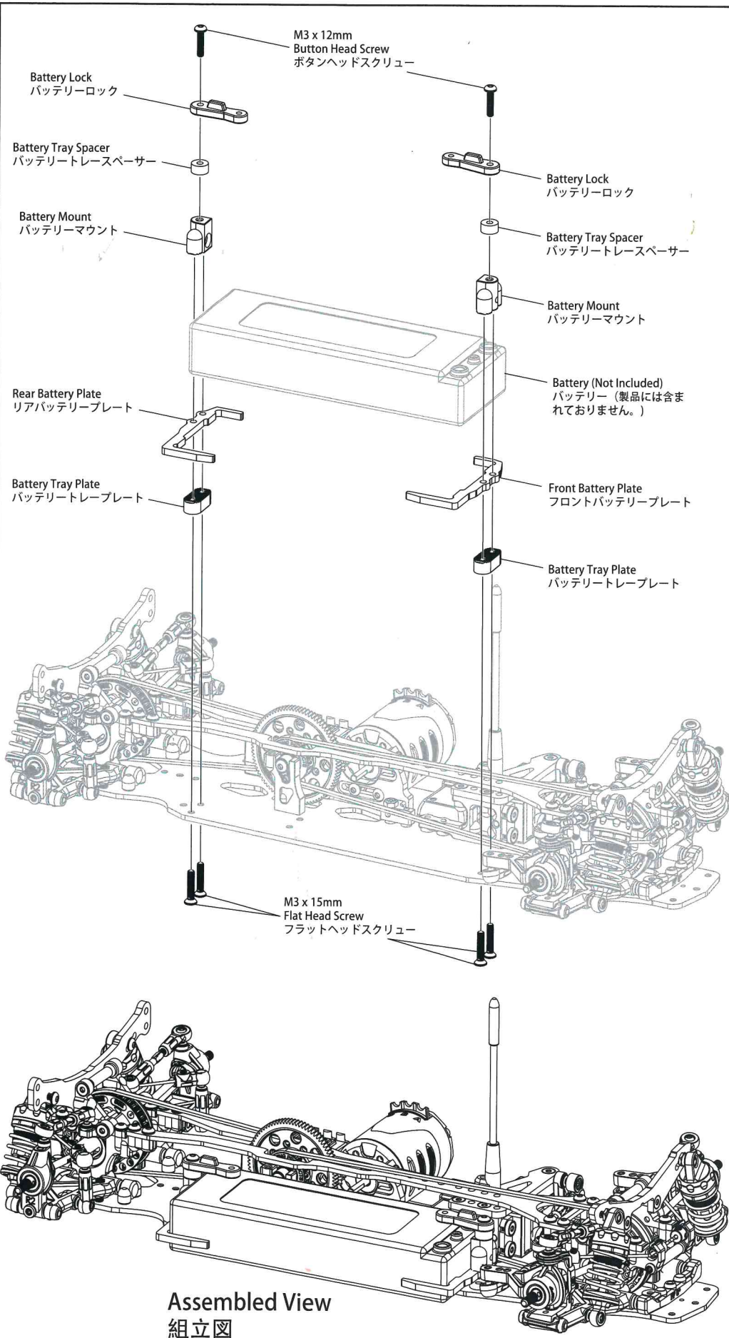
M3 x 15mm Flat Head Screw (4) M3 x 15mm フラットヘッドスクリュー (4)
