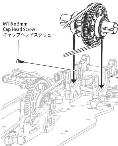
Default Belt Tension Setting 既定ベルトテンション設定
