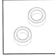
3RB-MR85-ZZ/W3/2 ¥25 Double Metal Shield Bearing 5 x 8 x 3mm (2 pcs) ダブルメタルシールドベアリン グ 5 x 8 x 3mm (2個入り)
