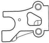
Center Pulley Mount - L (1) センタープーリーマウント - 左側 (1)
