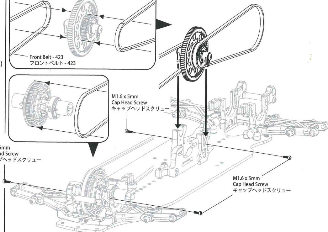
Bearing Holder - B ベアリングホルダー - B
