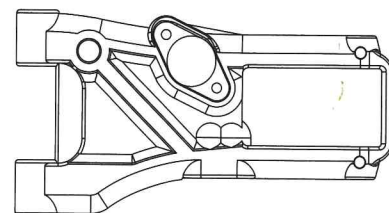
Front Suspension Arm (2) フロントサスアーム (2)
