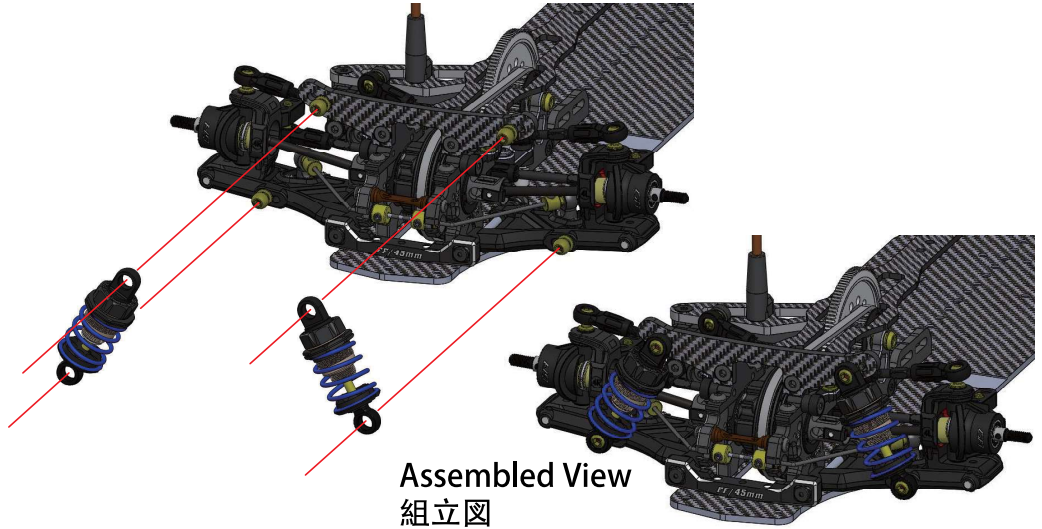
Aluminium Spring Base Cover 13mm アルミスプリングベースカバー-13mm
