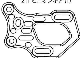
Motor Plate (1) モータープレート (1)
