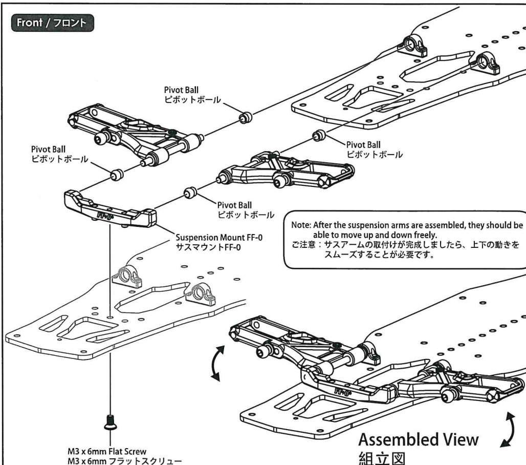
M3 x 6mm Flat Screw (2) M3 x 6mm フラットスクリュー (2)
