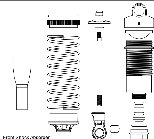
Front Shock Absorber 前避震器 2Set
