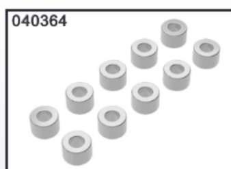
ALU WASHER 3X6X4
